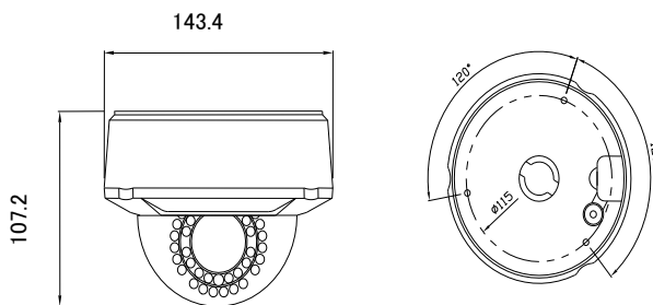
DIMENSION ( Unit : mm )
